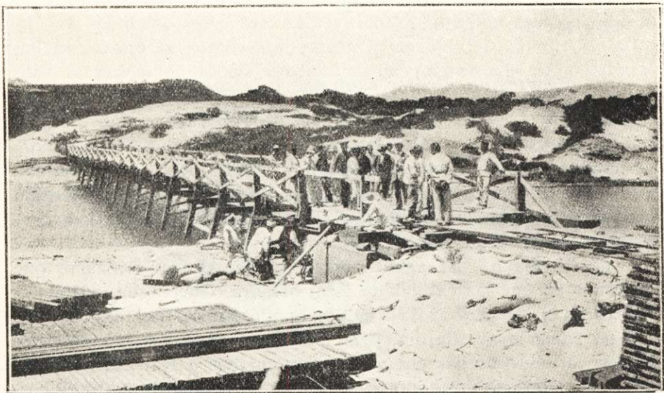
Puente sobre el río Negrón, construido por los ingenieros militares
