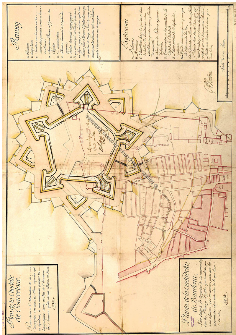
FIG. 9. Jorge Próspero Verboom (et al.), Plan de la Citadelle de Barcelone Pour servir a l'Adjudication de sa Construction avec toutes les Pièces séparées qui en dependent, Et sont nécessaires pour que les Entrepreneurs soient au fait de l'Execution des Travaux qu'ils seront obligés de faire | Planta de la Ciudadela de Barcelona, para servir á la Execucion de su construccion Con los Planos y Perfiles particulares, que van adjuntos, y se necesitan, para que los asentistas esten enterados de lo que han de Executar: Barcelona, ca. verano-otoño de 1715. Archivo General d Simancas. MPD, 10,051.
