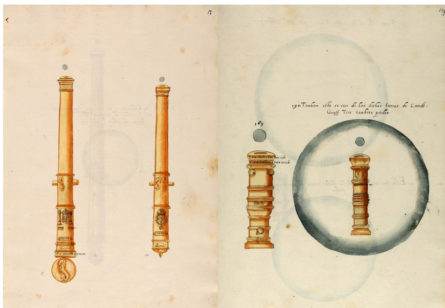
FIG. 2. Piezas de artillería fundidas para el emperador Carlos V por G. Löffler (ca. 1546) y pedreros requisados al landgrave Felipe I de Hesse tras la batalla de Mühlberg en 1547, en Jan Vredeman de Vries, Discurso del Artilleria del Invictissimo Emperador Carolo V , 1587. Mss. Universitätsbibliothek Erlangen-Nürnberg, H62/MS 2108, 12r y 139r, respectivamente.
