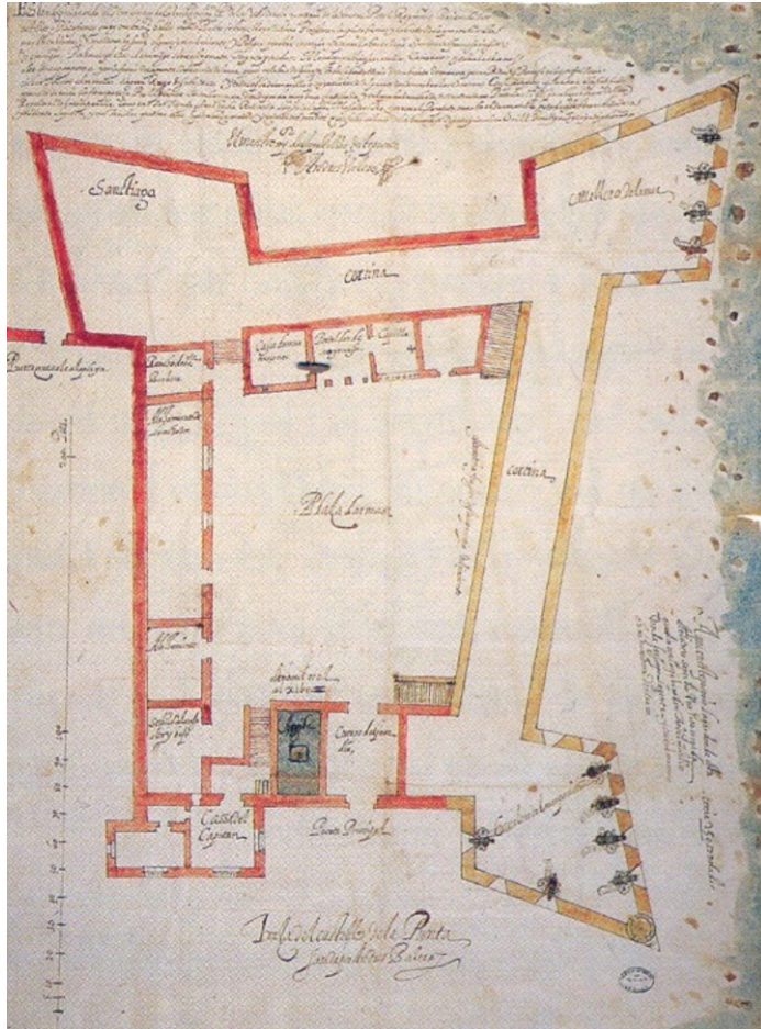
FIG. 9. Cristoforo Roda (Cristóbal de Roda), Castillo de la Punta de la Habana , 1595. Archivo General de Indias, M. y P., Santo Domingo, 16.
