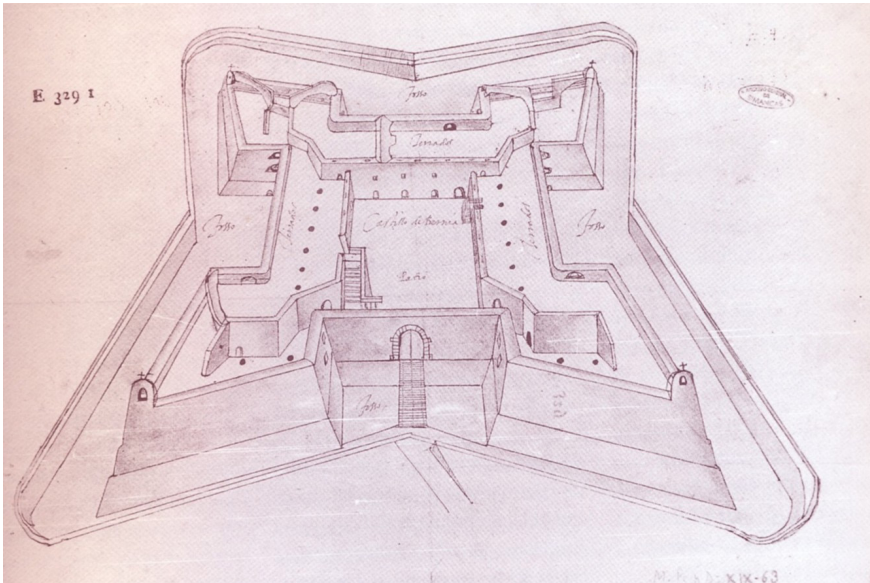
FIG. 4. Giovan Battista Antonelli (atribuido), Fortaleza de Bernia , 1563. Archivo General de Simancas, M.P. y D., XIX-63..
