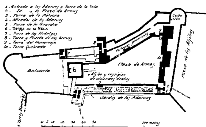
PLANO DE LA ALCAZABA DE LA ALHAMBRA
