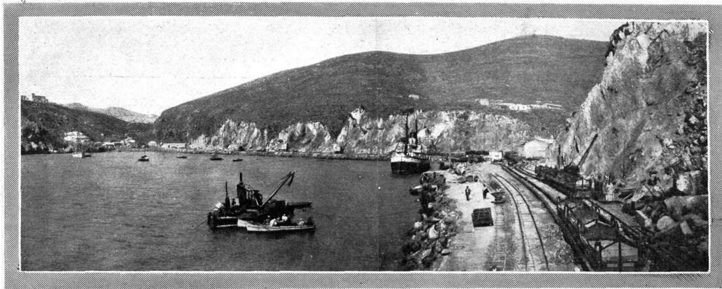
Estado actual de las obras del Puerto de Villa Sanjurjo.
