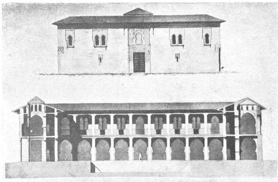
Hospital árabe de Granada - Fachada y sección
