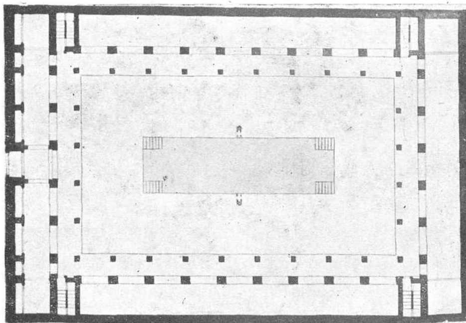
Hospital árabe (Moristán) de Granada - Planta
